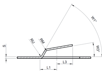
Z-linguetta / Z-Lasche
