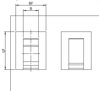
con pre-trancio / mit Freistanzung
