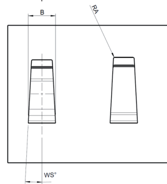
senza pre-trancio / ohne Freistanzung
